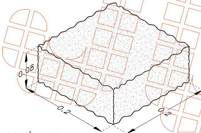
ISOMÉTRICO - Cotas en Metros
