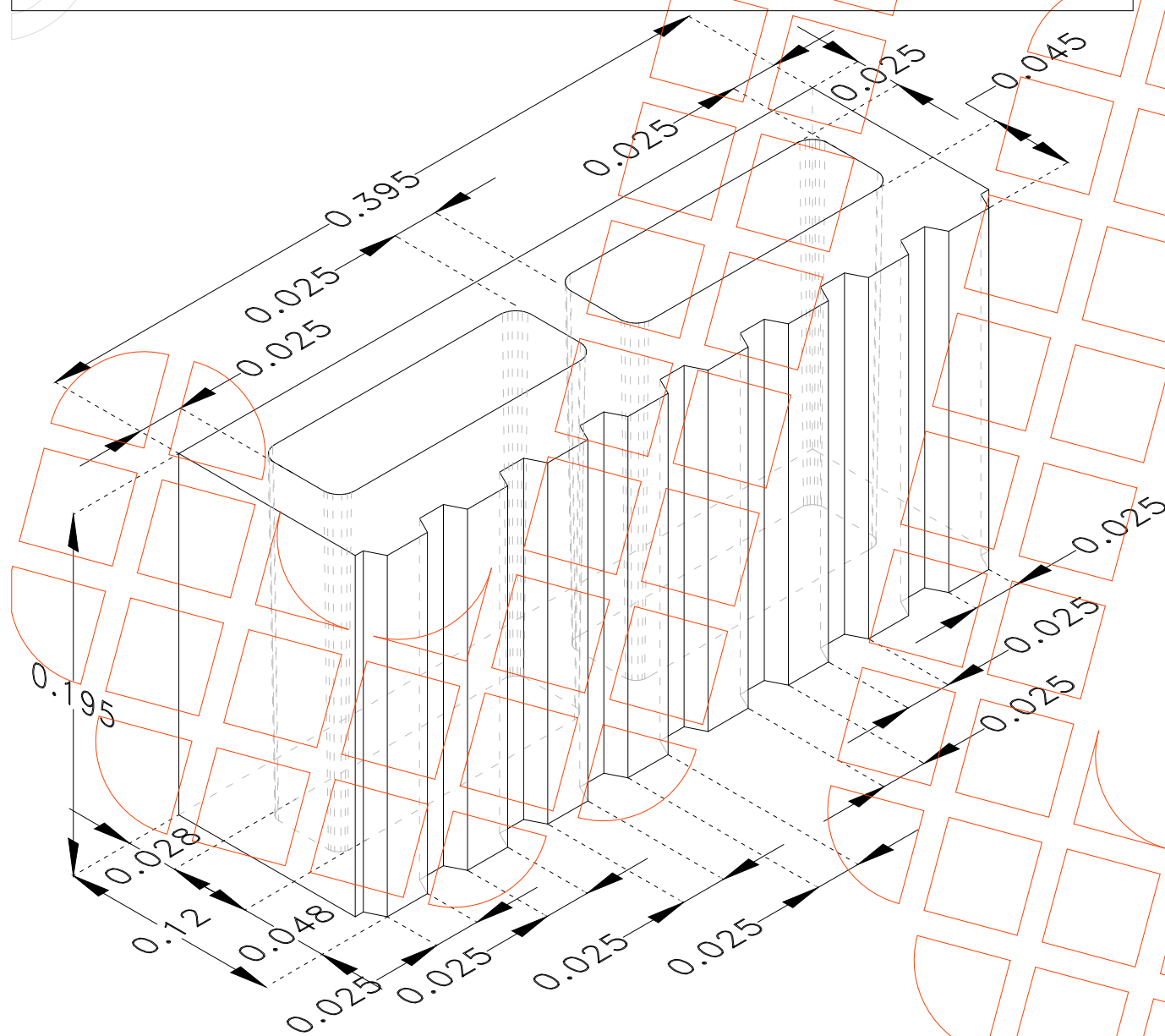
ISOMÉTRICO - Cotas en Metros
