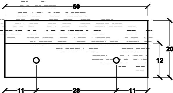
PLANTA
