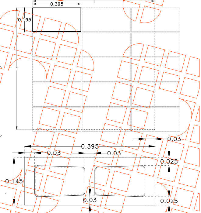
PLANTA - Cotas en Metros
