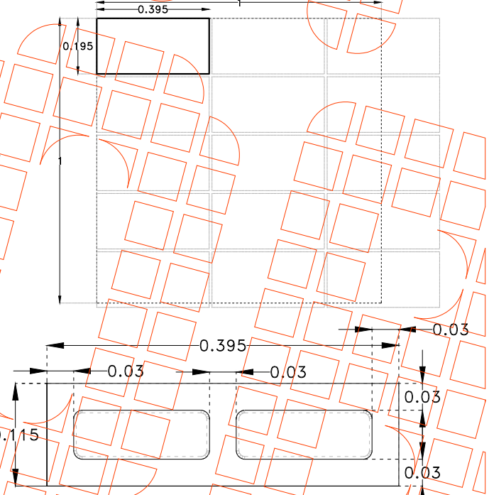
PLANTA - Cotas en Metros
